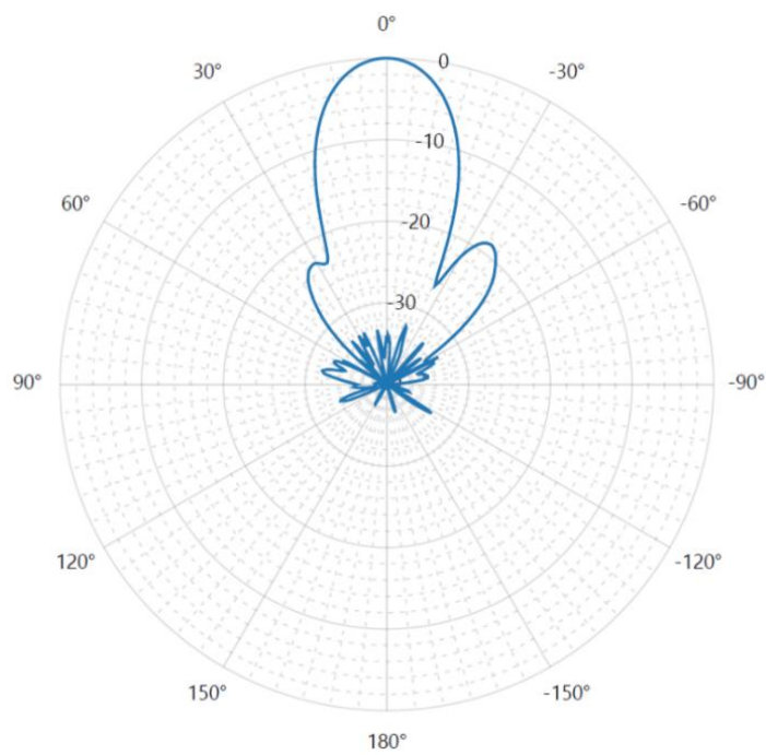
60 kHz 22° @ -3db
